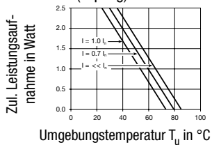
G-Sicherungseinsätze 5 x 20 mm (1-polig)
